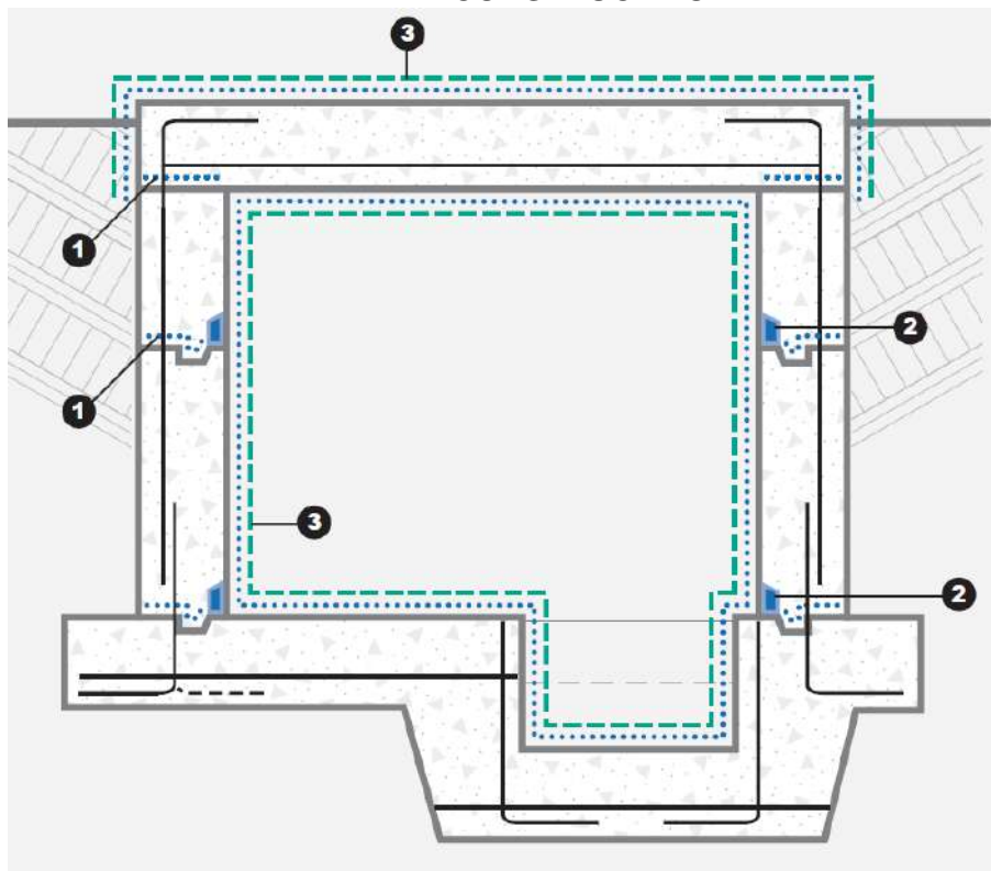
DETALLE CONSTRUCTIVO.
